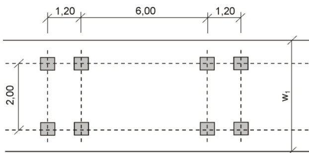
Obrázok P 2.16 Únavový zaťažovací model FLM3
