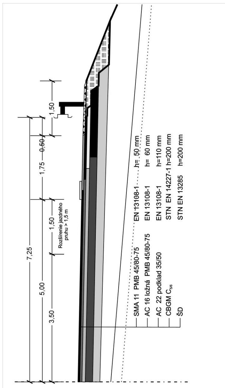
Obrázok 1 Priečny rez rozšírenia vozovky
