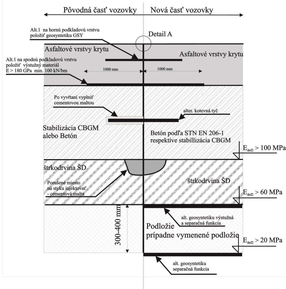
Obrázok 2 Schéma rozšírenia vozovky o jazdný pruh detail priečného rezu
