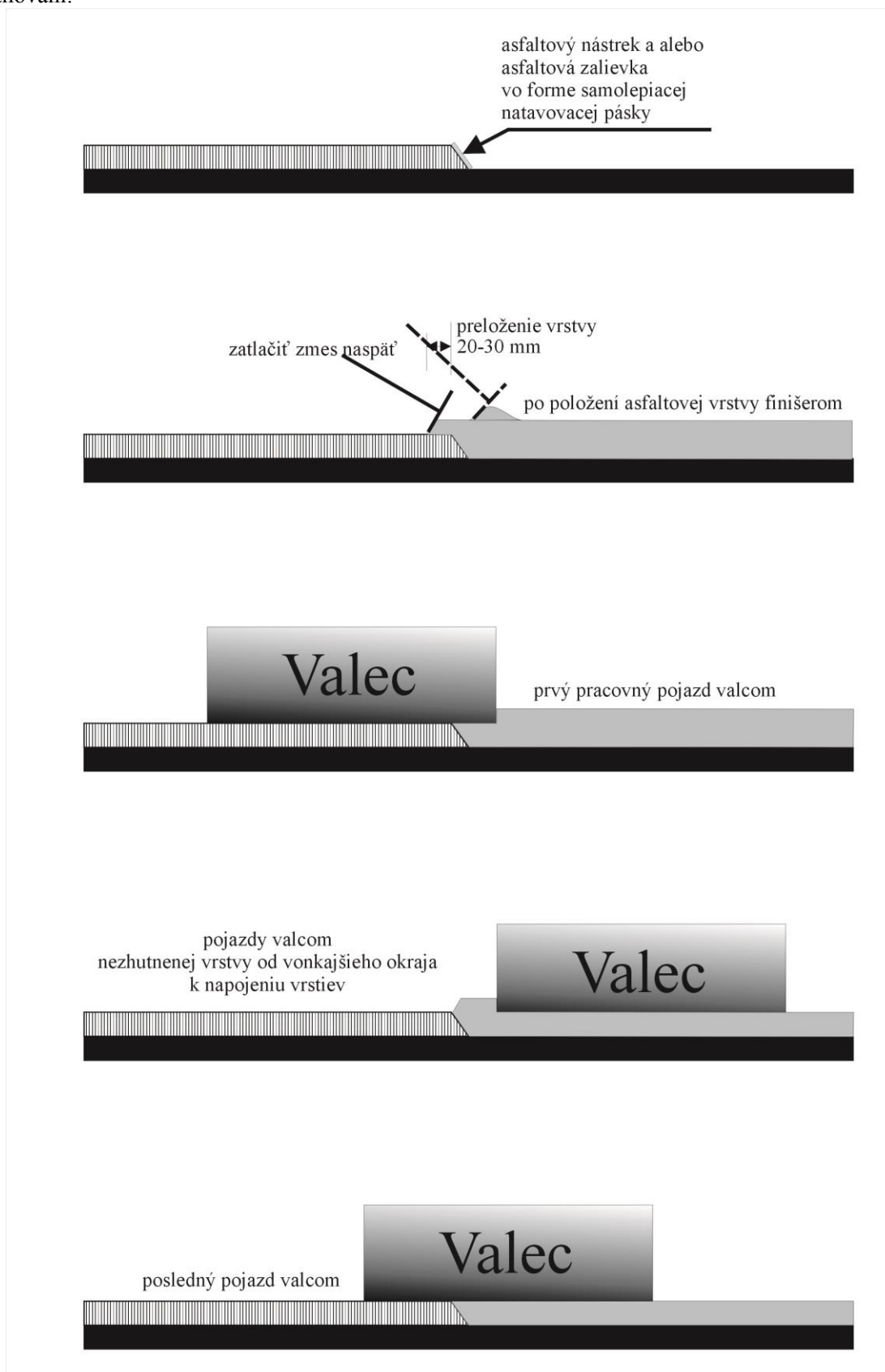
Obrázok 4 Technologický postup napájania asfaltových zmesí pri zhutňovaní
