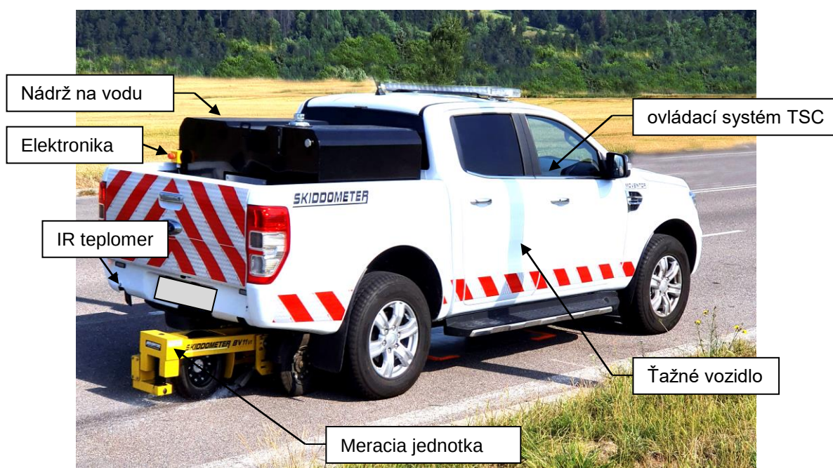
Obrázok 1 Zariadenie Skiddometer BV 11 VI
