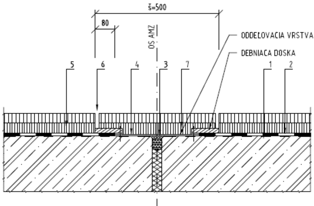
Obrázok 9 - Základný postup zhotovenia vybratia v novej vozovke
